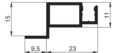
10 23 04 Spannrahmenprofil
