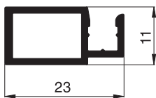
10 23 02 Spannrahmenprofil
