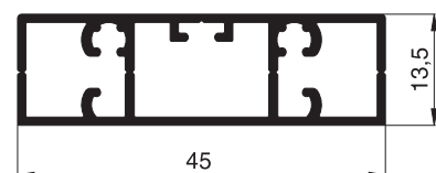
10 42 12 unteres Montagerahmenprofil
