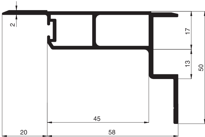
10 32 14 Lichtschachtdeckungsprofil
