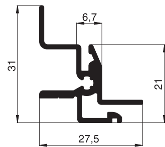
10 33 22 Adapterprofil
