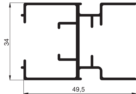
10 42 05 bewegliches Flügelprofil
