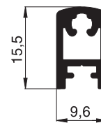
10 39 21 unteres Rahmenprofil
