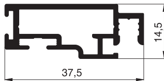
10 35 06 Drehrahmenprofil
