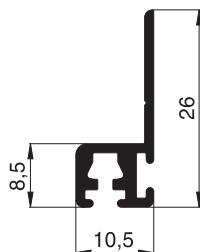
10 35 61 h-Profil
