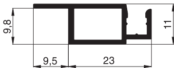
10 23 05 Spannrahmenprofil
