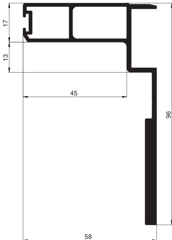
10 32 18 Statikprofil
