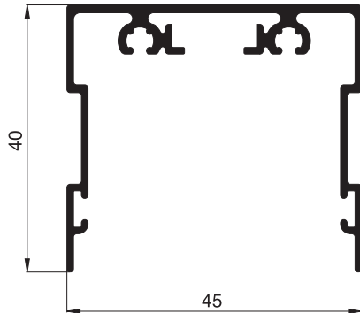
10 42 01 Kastenprofil
