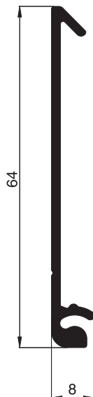
10 43 12 Kastenblendenteil vorne
