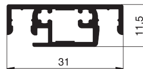
10 35 11 Sprossenprofil
