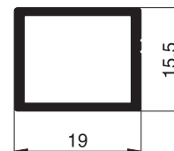
10 35 22 Montagerahmenprofil
