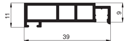
10 24 52 Spannrahmenprofil
