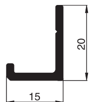
10 43 91 Montageprofil
