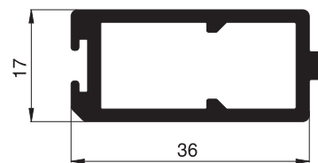
10 32 40 Adapterprofil
