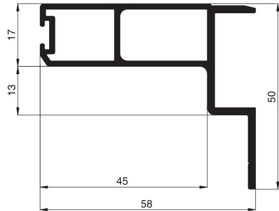
10 32 16 Lichtschachtdeckungsprofil
