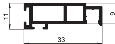
10 24 06 Spannrahmenprofil
