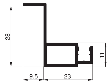
10 23 07 Spannrahmenprofil
